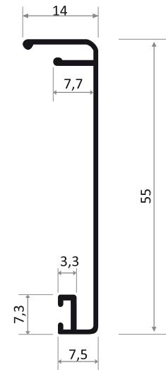
AF - 45 Trilho Inferior pesado
