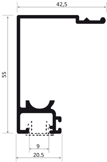
AF - 50AL Capa p/ Trilho Superior 6,10 mm
